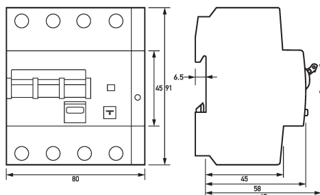
Maßzeichnung Gruppenansicht
