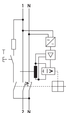
Schaltungsbeispiel FI-/LS-Kombinationen DRCBO 4 B32/0,30/1N-B NK
