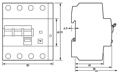
Maßzeichnung FI-/LS-Kombinationen DRCBO 4 B25/0,10/3N-B NK
