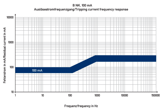
Diagramme FI-/LS-Kombinationen DRCBO 4 B25/0,10/3N-B NK
