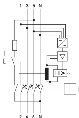
Schaltungsbeispiel FI-/LS-Kombinationen DRCBO 4 B25/0,10/3N-B NK
