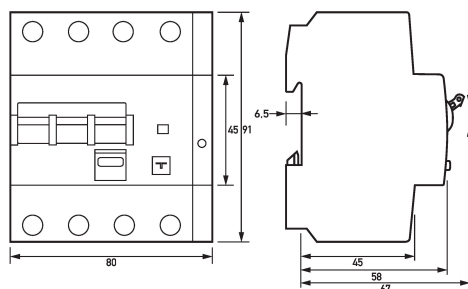
Maßzeichnung FI-/LS-Kombinationen DRCBO 4 B20/o,30/3N-B NK
