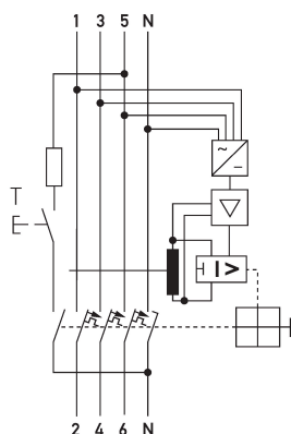
Schaltungsbeispiel FI-/LS-Kombinationen DRCBO 4 B20/o,30/3N-B NK
