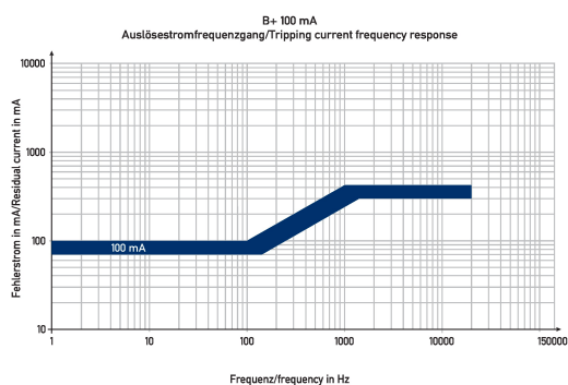
Diagramme FI-/LS-Kombinationen DRCBO 4 B20/0,10/1N-B+
