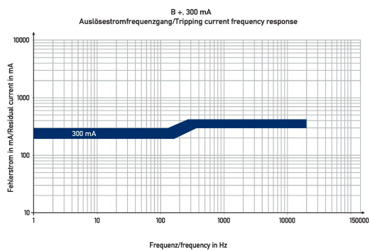
Diagramme FI-/LS-Kombinationen DRCBO 4 B13/0,30/3N-B+
