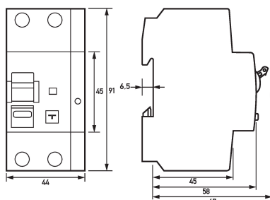
Maßzeichnung Gruppenansicht
