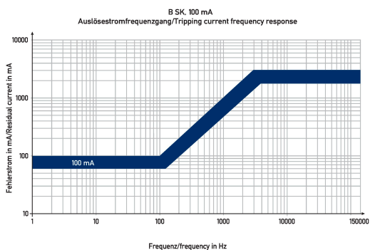
Diagramme FI-/LS-Kombinationen DRCBO 4 B10/0,10/1N-B SK
