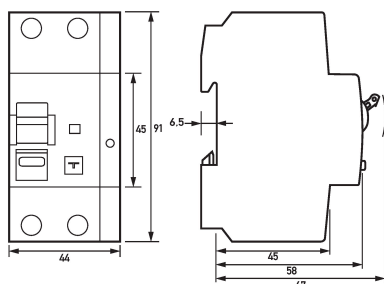
Maßzeichnung FI-/LS-Kombinationen DRCBO 4 B10/0,10/1N-B SK
