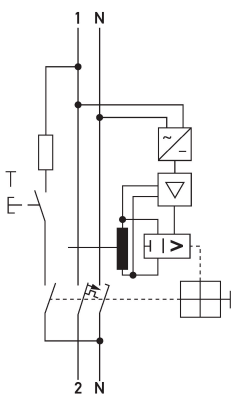
Schaltungsbeispiel FI-/LS-Kombinationen DRCBO 4 Bo6/0,10/1N-B NK
