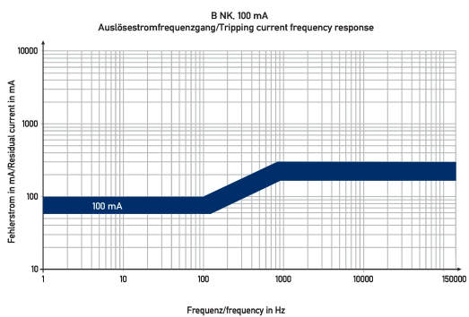
Diagramme FI-/LS-Kombinationen DRCBO 4 Bo6/0,10/1N-B NK
