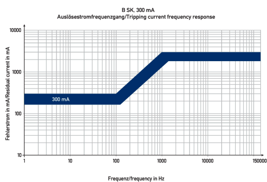
Diagramme FI-/LS-Kombinationen DRCBO 4 B32/0,30/1N-B SK
