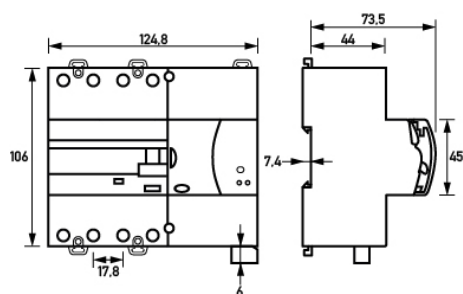
Maßzeichnung Gruppenansicht
