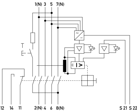
Anschlusschema
