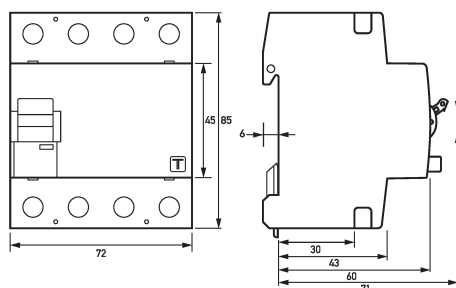
Maßzeichnung Fehlerstromschutzschalter DFS 4 063-4/0,50-A R
