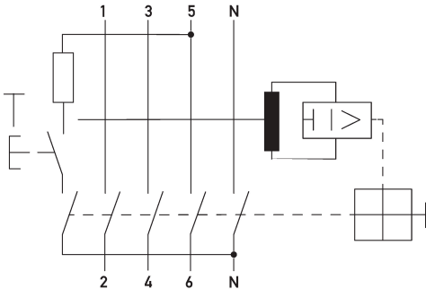
Schaltungsbeispiel Fehlerstromschutzschalter DFS 4 040-4/0,50-A R
