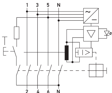
Schaltungsbeispiel Fehlerstromschutzschalter DFS 4 040-4/0,30-B SK R HD
