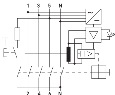
Schaltungsbeispiel Fehlerstromschutzschalter DFS 4 040-4/0,03-B SK R ISO HD
