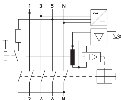
Schaltungsbeispiel Fehlerstromschutzschalter DFS 4 025-4/0,30-B SK R HD
