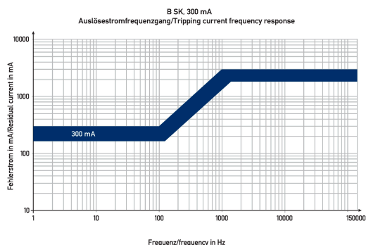
Diagramme Fehlerstromschutzschalter DFS 4 025-4/0,30-B SK HD
