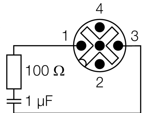
Anschlussbild
