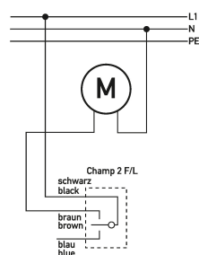
Schaltungsbeispiel Schwimmerschalter Champ 2 G-L/F 03 m
