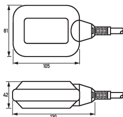
Maßzeichnung Schwimmerschalter Champ 2 G-L/F 03 m
