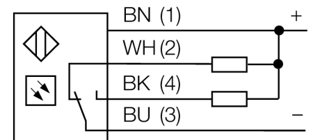
Anschlussbild
