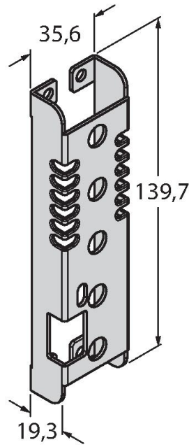
SMBPVA1
