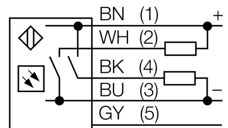
Anschlussbild
