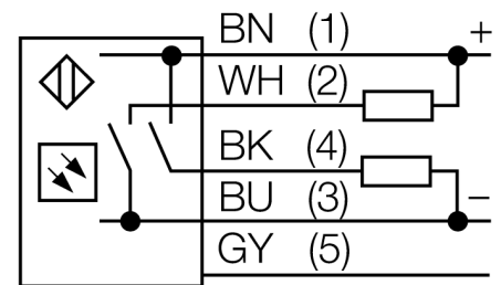
Anschlussbild
