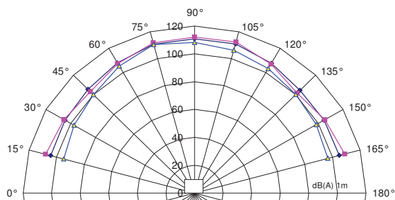
DS 10 puissance sonore - diagramme vertical
