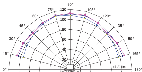
DS 10 Schallpegel Vertikaldiagramm
