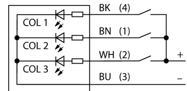
Anschlussbild
