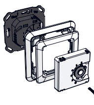
Regler 50 x 50 mit Beispiel-Rahmen und Zwischenrahmen
