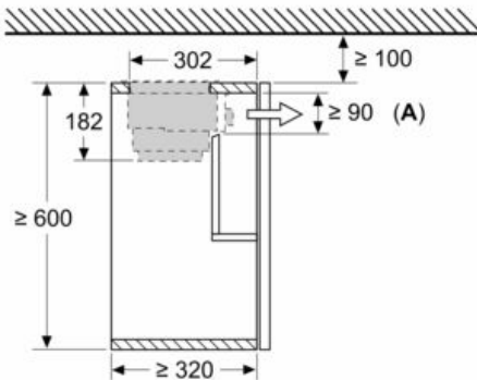
Maße in mm Montage Flachschildhaube mit Umluftset
