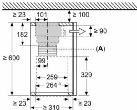
Maße in mm Montage Lüfterbaustein mit Umluftset
