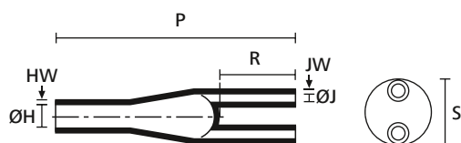
b: Formteil nach vollständiger Schrumpfung
