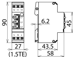
Maßbild DSI E 3
