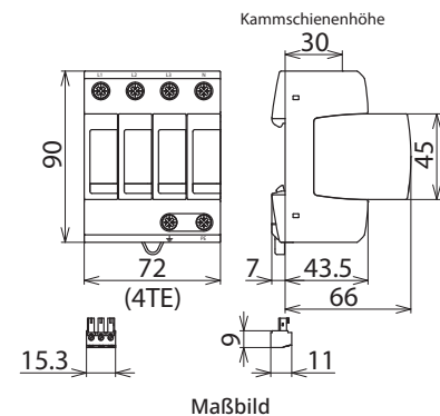
Maßbild
