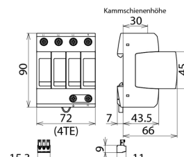
Maßbild DG M TT 385 FM
