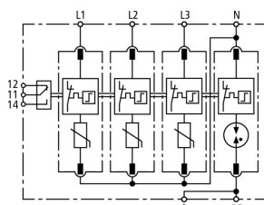
Prinzipialschaltbild DG M TT 385 FM
