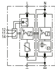
Prinzipschaltbild DG M TT 2P ACI 385 FM
