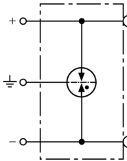
Prinzipschaltbild BT 24
