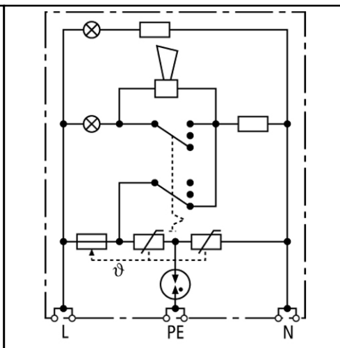
Prinzipschaltbild DSA 230 LA
