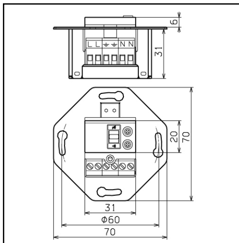
Maßbild DSA 230 LA
