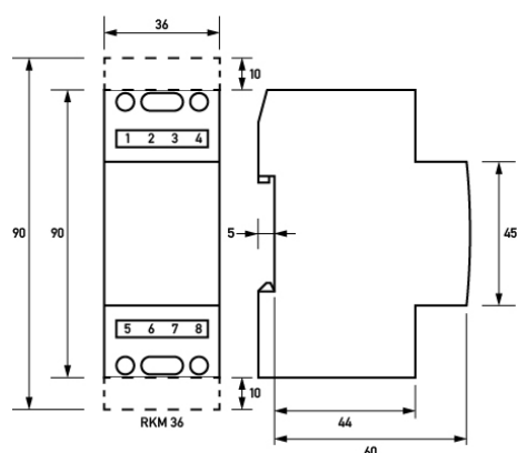
Maßzeichnung Gruppenansicht
