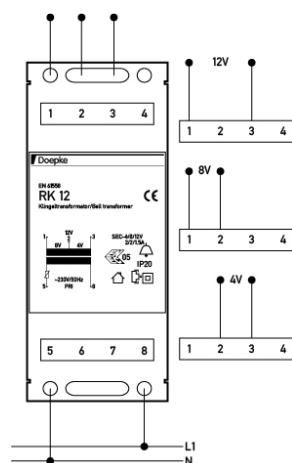
Anschlusschema
