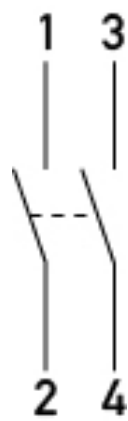
Anschlusschema
