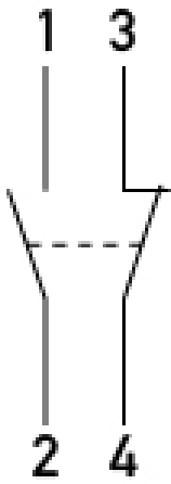
Anschlusschema
