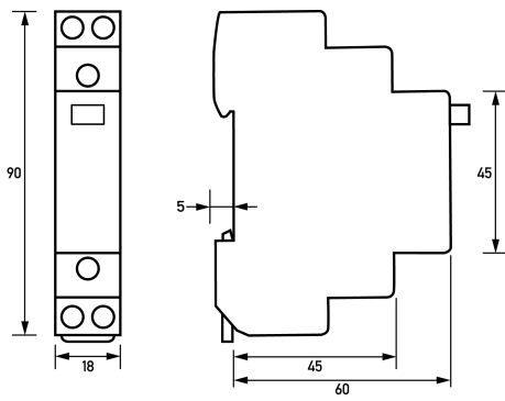
Maßzeichnung Gruppenansicht
