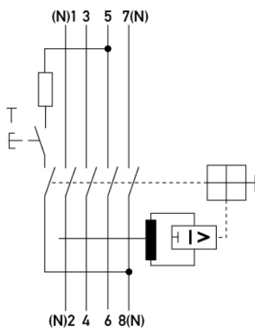
Anschlussschema
