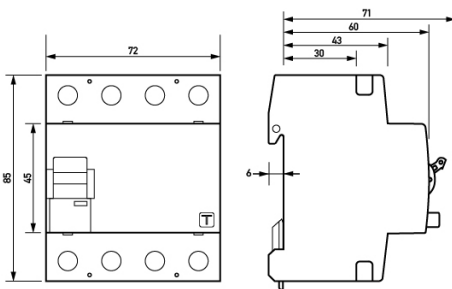
Maßzeichnung Gruppenansicht
