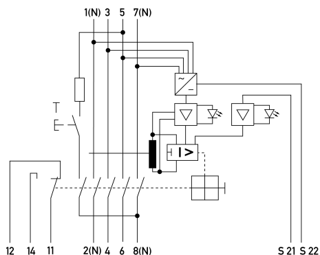
Anschlusschema
