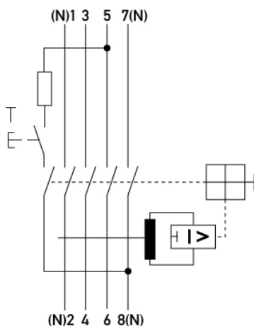
Anschlusschema
