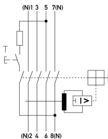
Anschlussschema
