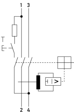
Anschlusschema
