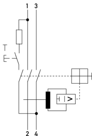
Anschlusschema
