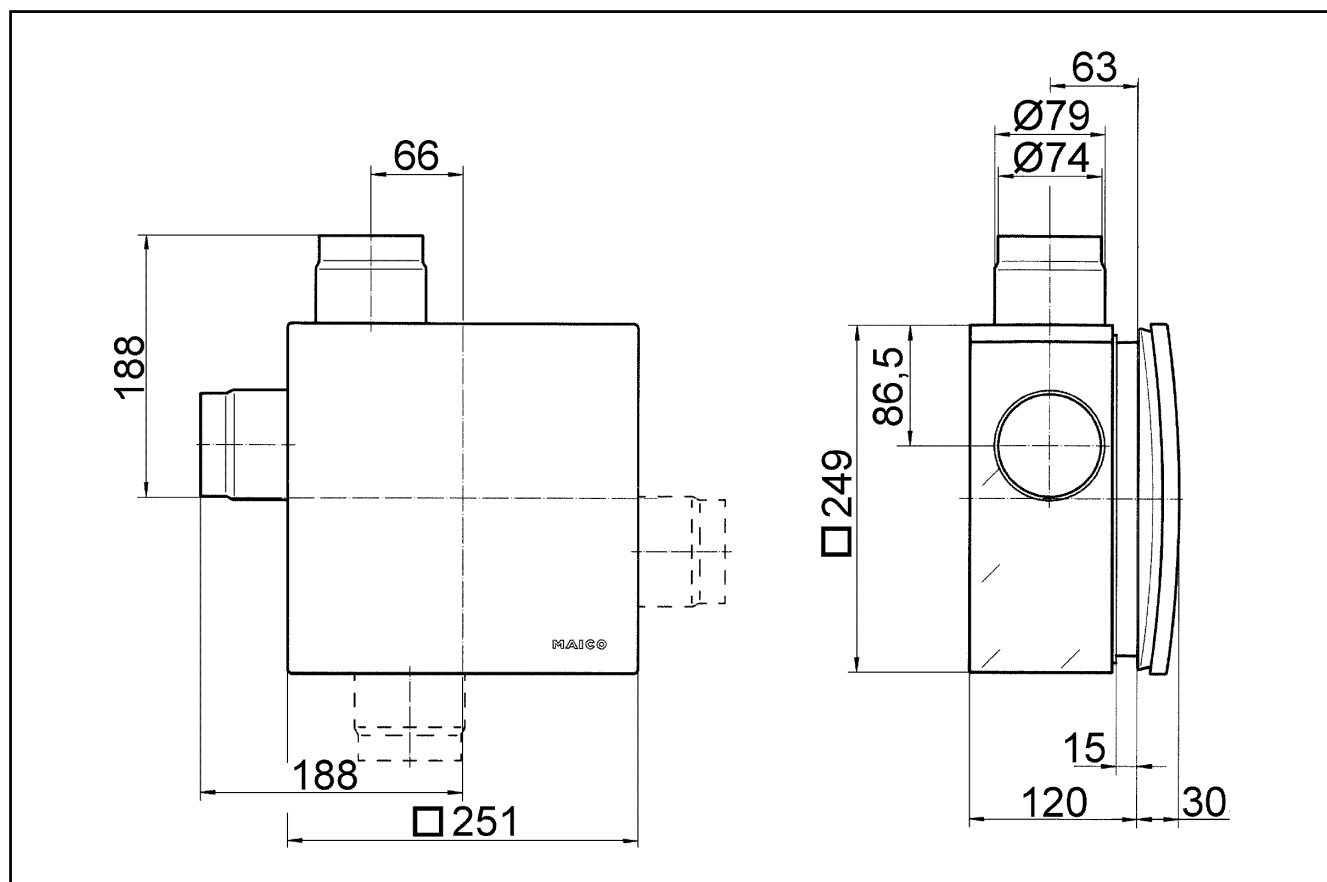
ER-UPB mit Zweitraumanschluss
