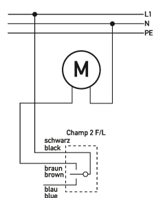
Schaltungsbeispiel Schwimmerschalter Champ 2 G-L/F 05 m
