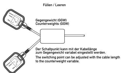
Anschlusschema
