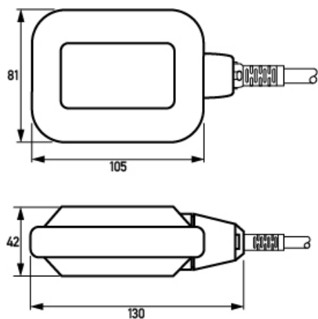
Maßzeichnung Gruppenansicht
